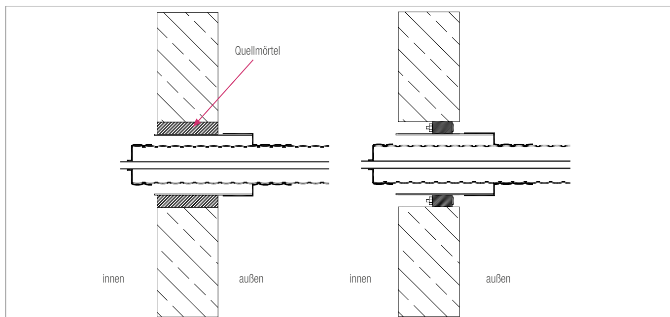
Abb. 3: Skizze Einbauvariante 1
