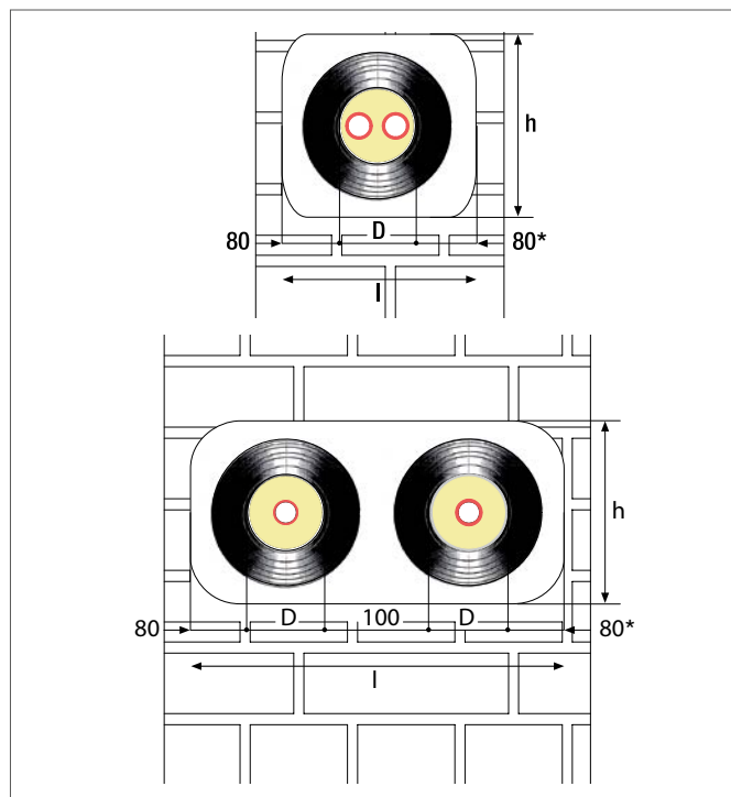
Abb. 2: Abmessungen Mauerdurchbruch UNO & DUO Rohr*
