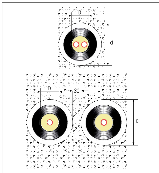
Abb. 3: Abmessung Kernlochbohrung UNO & DUO Rohr*
