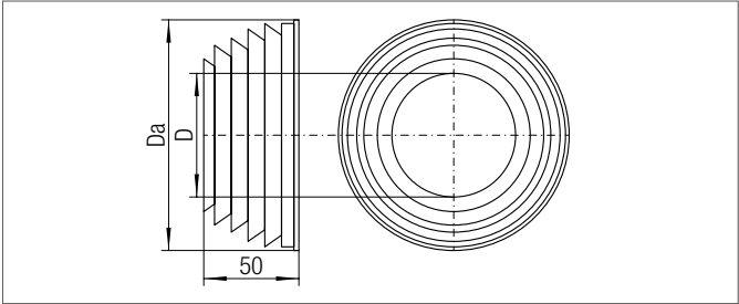
Abb. 1: Bemaßung des Dichtrings
