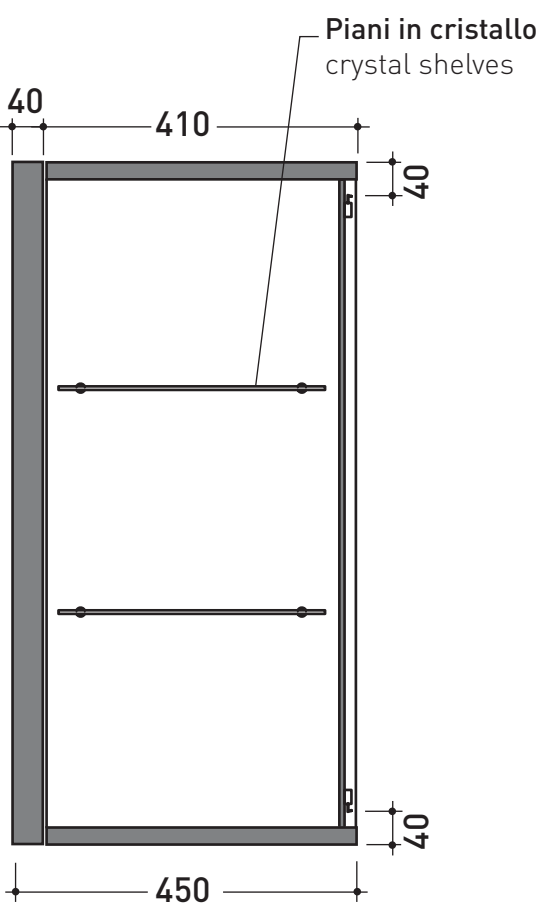
sezione longitudinale / section
