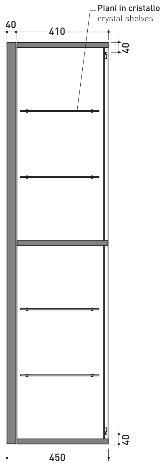
sezione longitudinale / section
