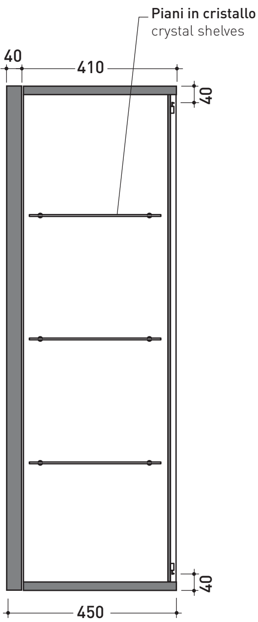
sezione longitudinale / section
