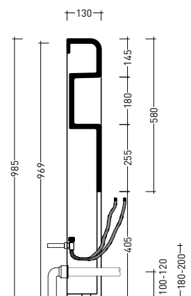
sezione / section
