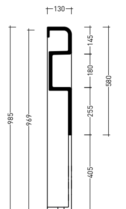
sezione / section
