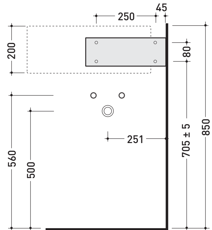
vista frontale fissaggio staffa fixing bracket frontal view
